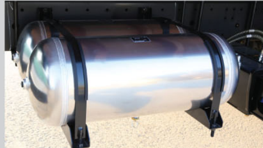
알루미늄 에어탱크
